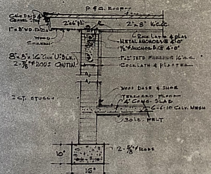
• WALL SECTION
