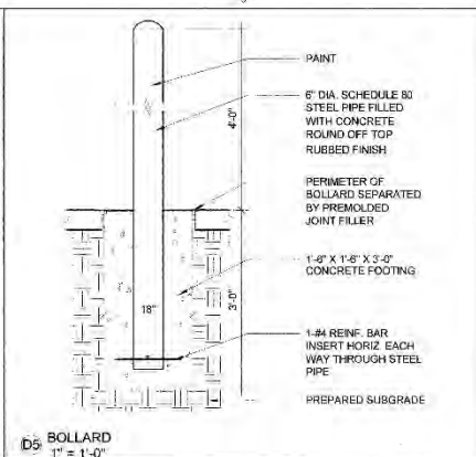
D5 BOLLARD 1" = 1'-0"
